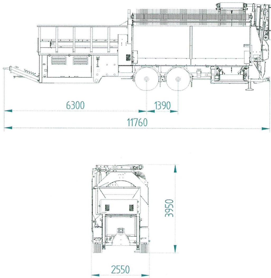
Afb. 6: Maattekening Trommelzeefmachine T 55 (transportstand)
