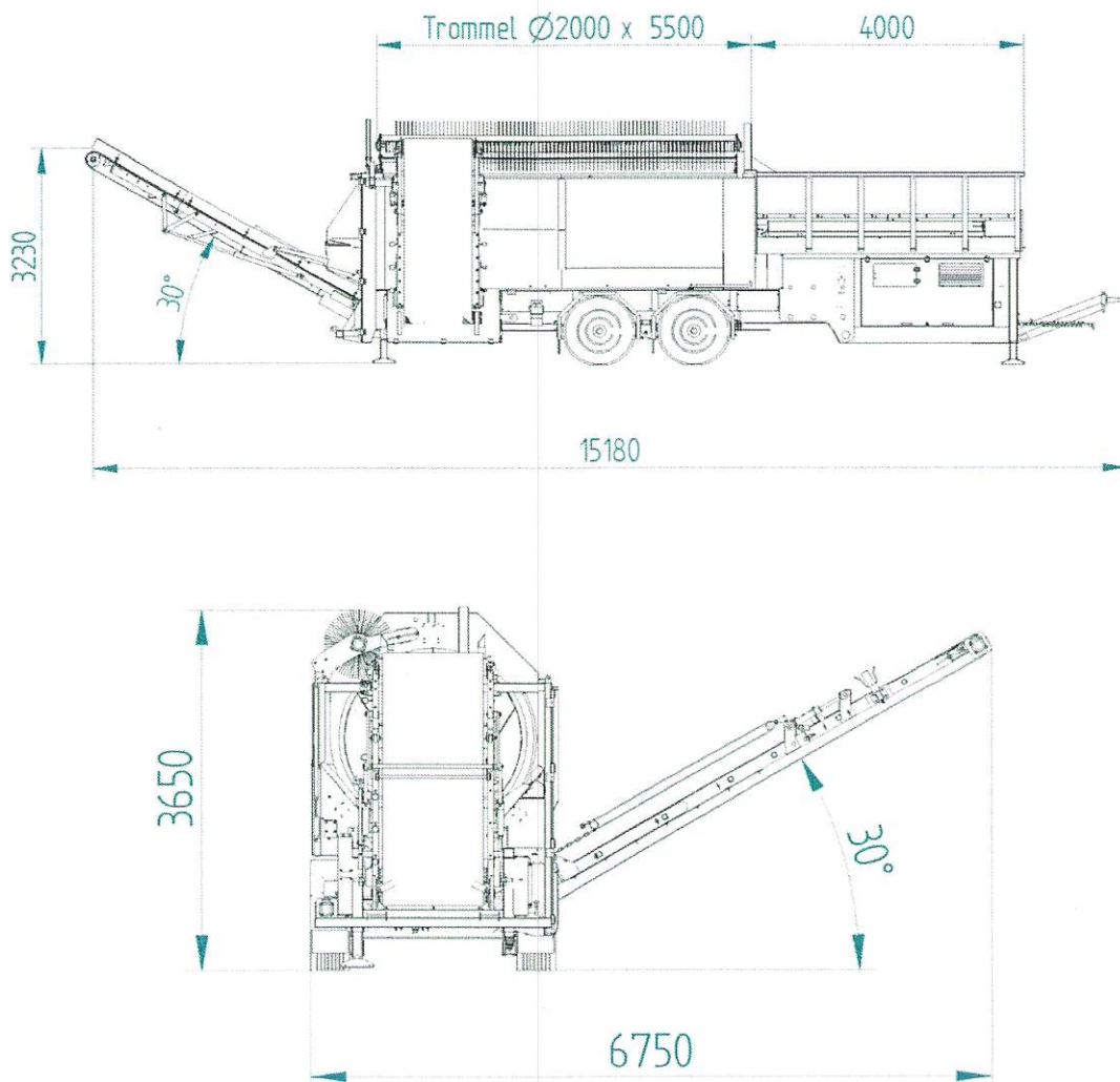
Afb. 7: Maattekening Trommelzeefmachine T 55 (werkstand)
